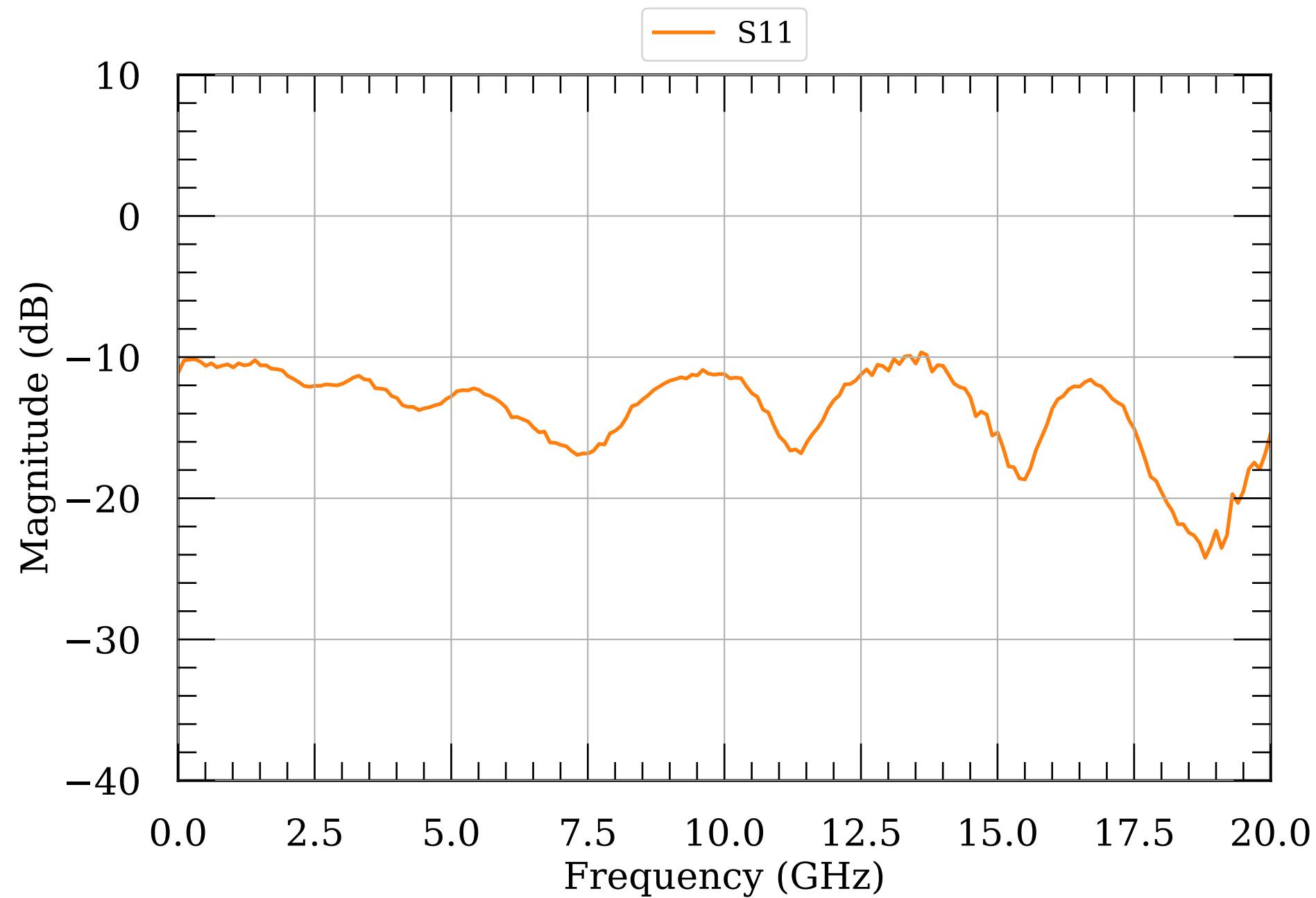
LNA S-params module069
